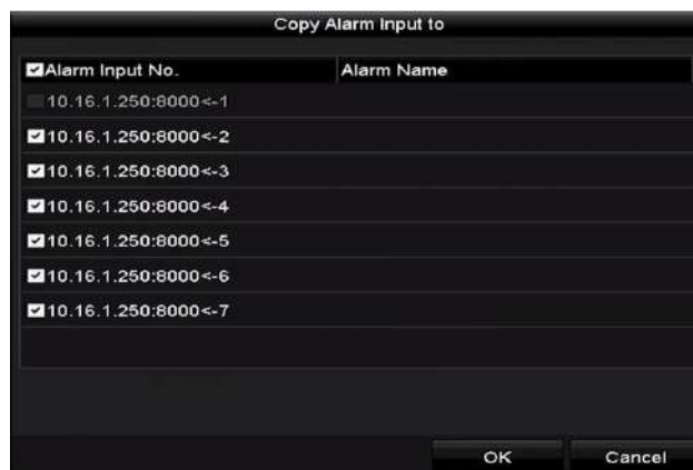
Рисунок 5-20 Копирование тревожного входа
