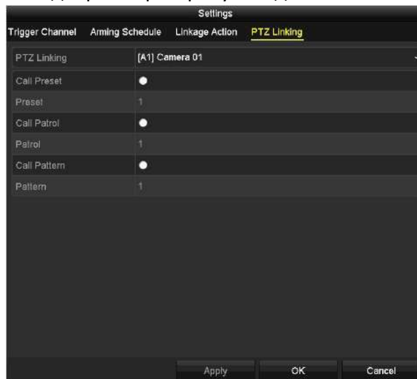
Рисунок 8-8 Привязка PTZ к тревожному входу
