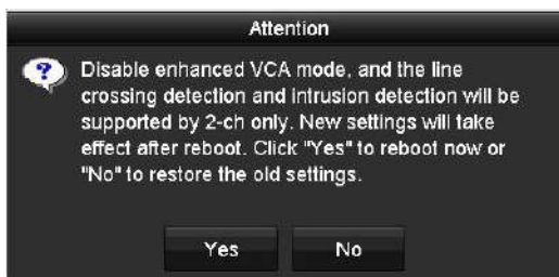
Рисунок 17-11 Отключение расширенного режима VCA
