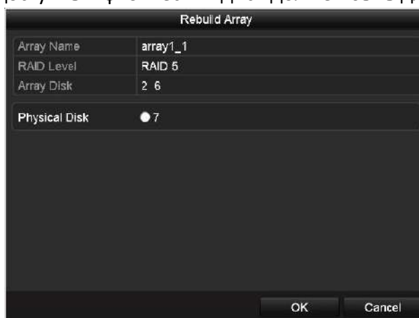
Рисунок 13-13 Меню перестройки массива
