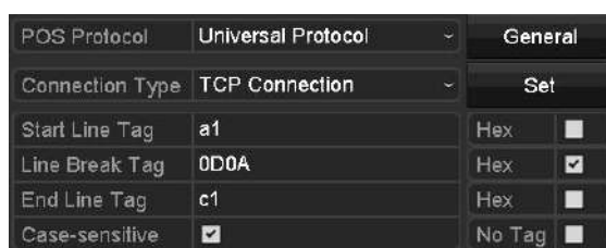
Рисунок 9-3 Настройки универсального протокола
