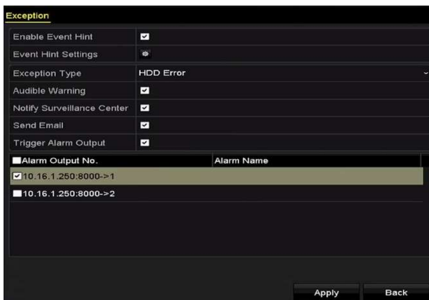
Рисунок 14-31 Настройка тревоги ошибки HDD
