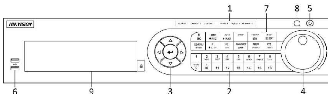
Рисунок 1-4 Передняя панель DS-8100HQHI-F/N и DS-8100HUNI-F/N
