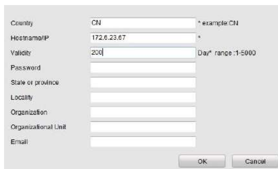
Рисунок 12-20 Создание самоподписанного сертификата
